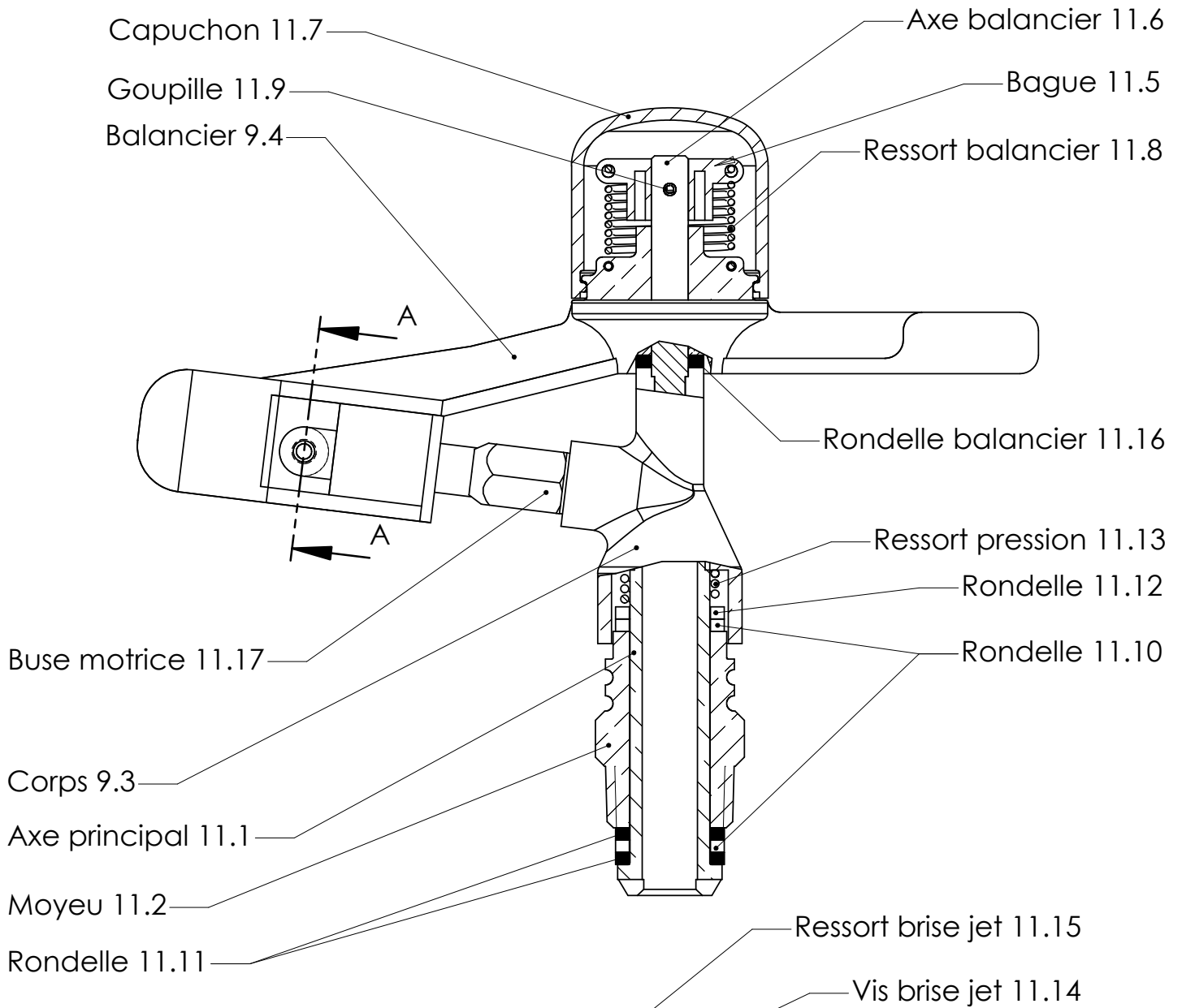
COUPE A-A
